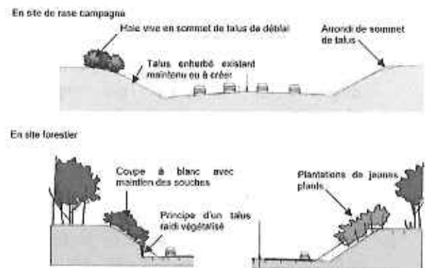
Figure 8 : coupe de principe sur le traitement des passages en déblais.
