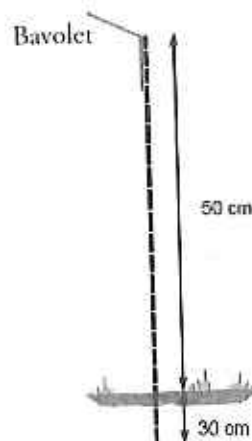
Figure 18 : Exemple de clôture - Source : J. Carsignol (CETE de l'Est) et E. Rillardon (Sétra)
