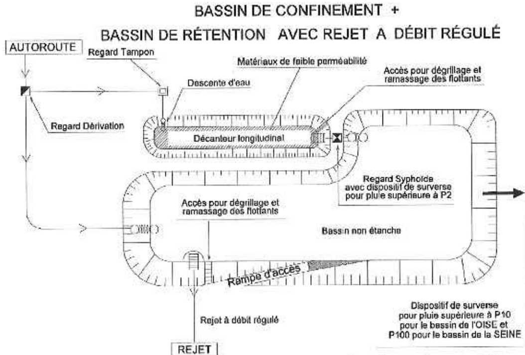
Figure 14 : schéma de principe du bassin de rétention et des de confinement des eaux de ruissellement de la plateforme autoroutière
