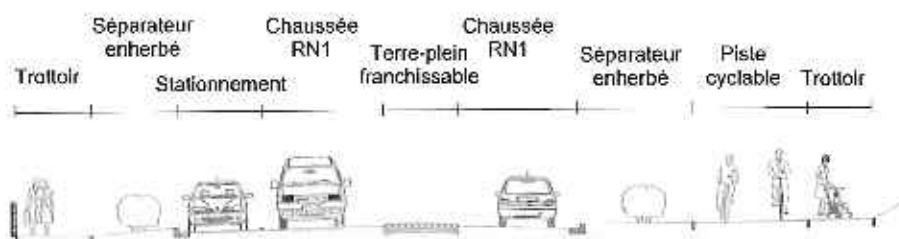
Figure 27: configuration routière envisagée au hameau de l'Orme aux Roses –schématisation Béture infrastructures
