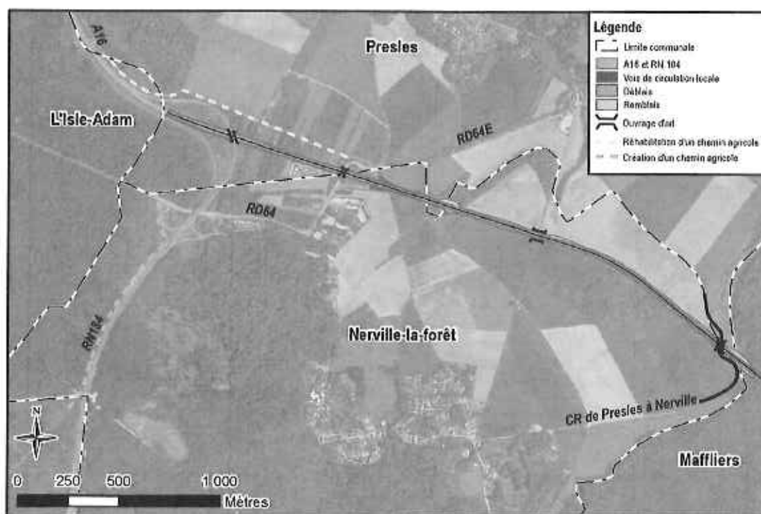
Figure 42 : rétablissement et réhabilitation des chemins agricoles dans la partie Nord du projet A16
