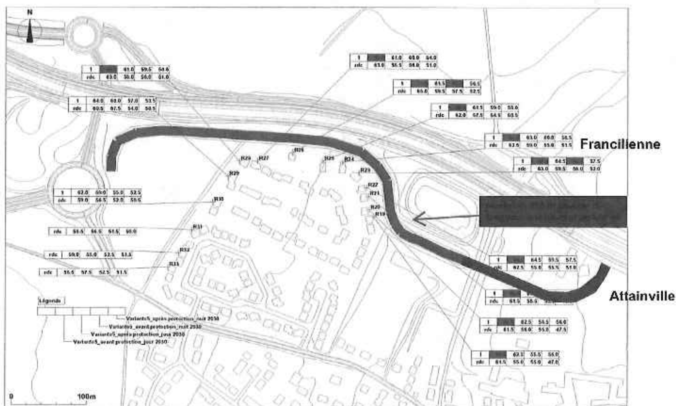
Figure 41 : prolongement du merlon acoustique au niveau d'Attainville
