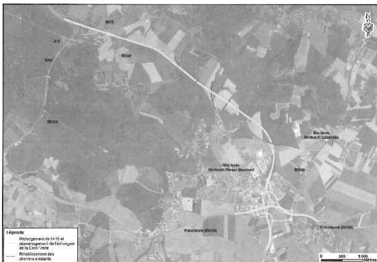
Figure 3 : tracé prévu du prolongement de l'A16
