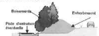
Figure 9 : coupe de principe sur le traitement des passages des merlons acoustiques.
