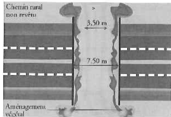
Figure 22 : exemple d'aménagement de passage à faune supérieur mixte
