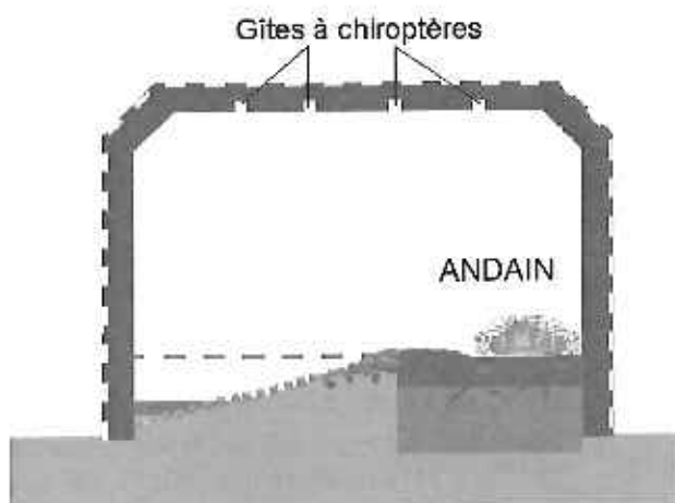
Figure 23 : schéma de principe de l'aménagement de l'ouvrage hydraulique du bois Carreau en passage faune
