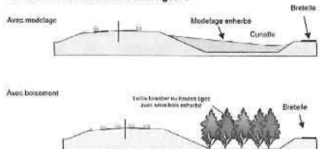
Figure 10: coupe de principe sur le traitement des boucles d'échangeurs.
